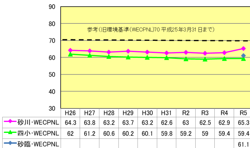
WECPNL 立川飛行場の航空機騒音 (WECPNL)
