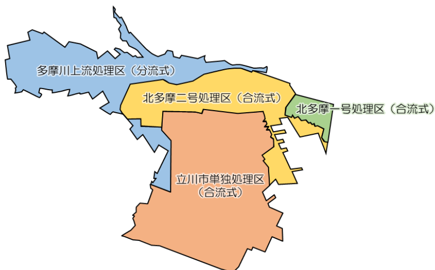
図 2-1 立川市の処理区
