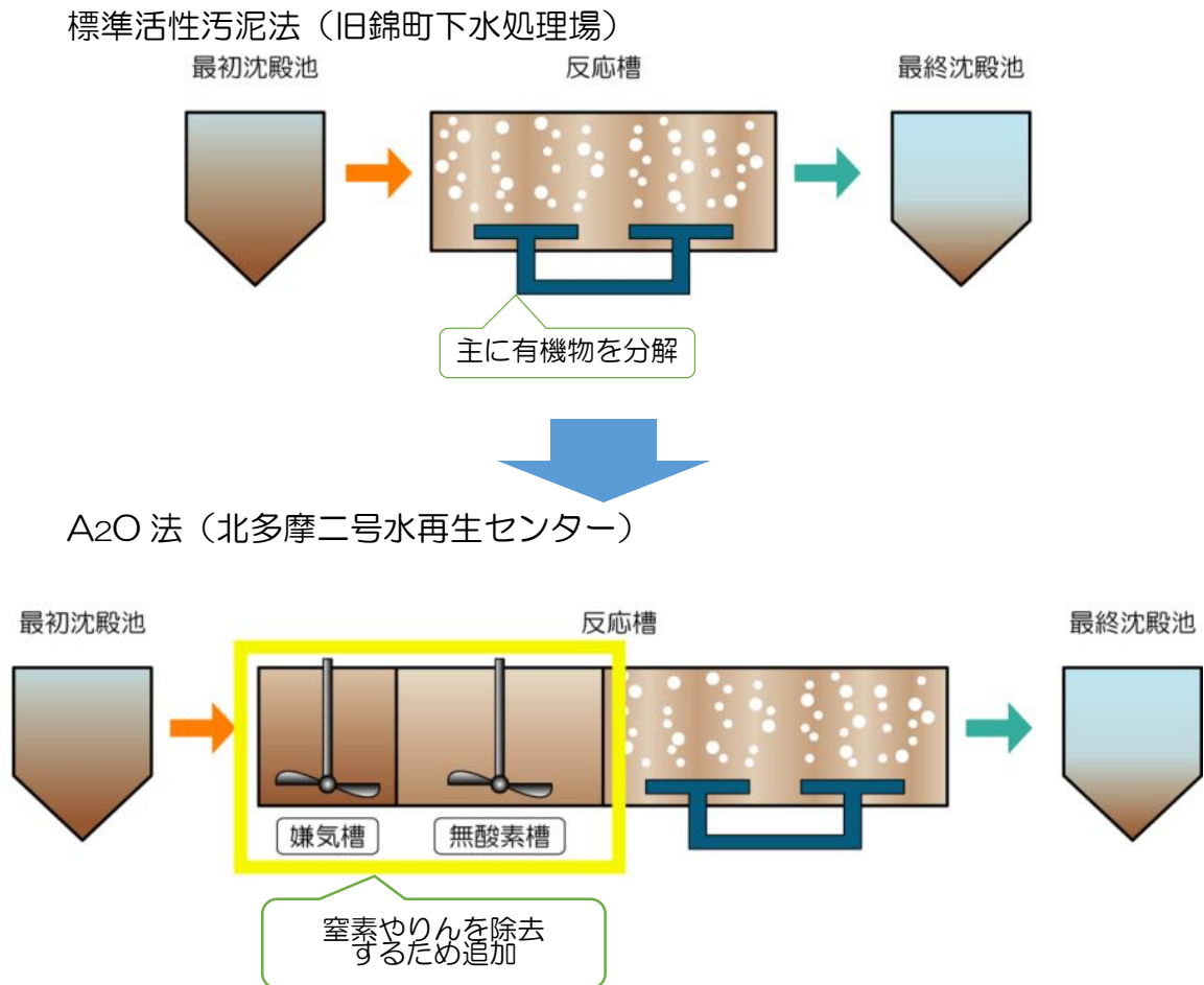
図3-7 処理方式の変更
