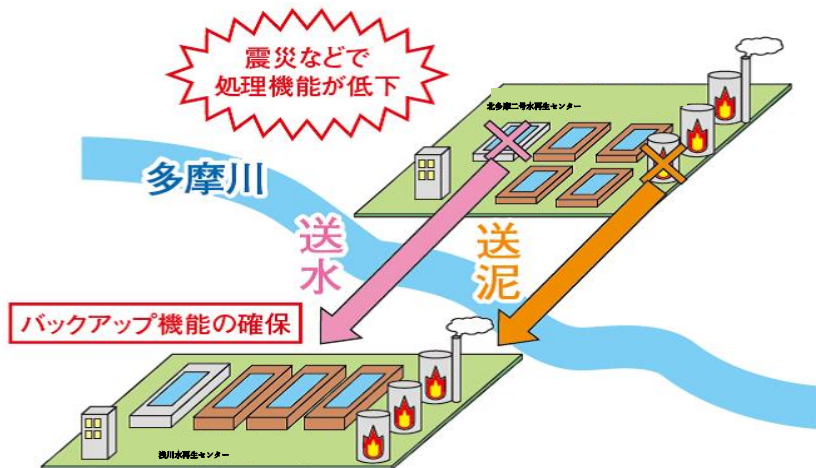
図3-8 連結管によるバックアップ機能
