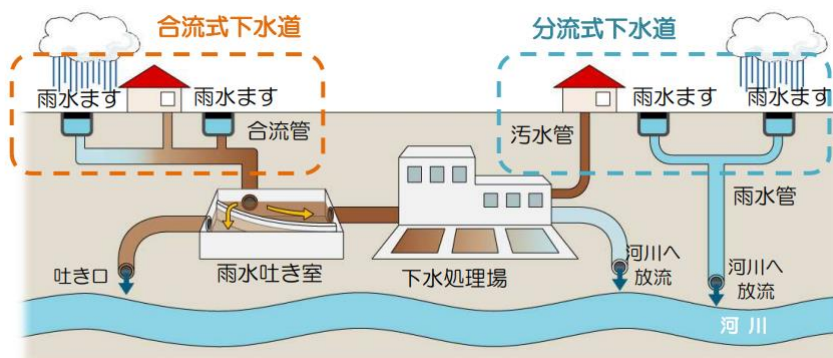
図 2-2 合流式下水道と分流式下水道
